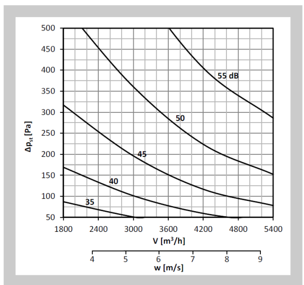
Diagram nr 58 Poziom mocy akustycznej LWA [dB(A)] na zewnątrz kanału 400x400, z izolacją
