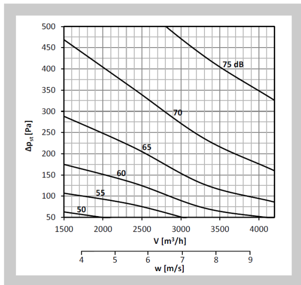
Diagram nr 11 Poziom mocy akustycznej L_{WA} [dB(A)] w kanale 400x300
