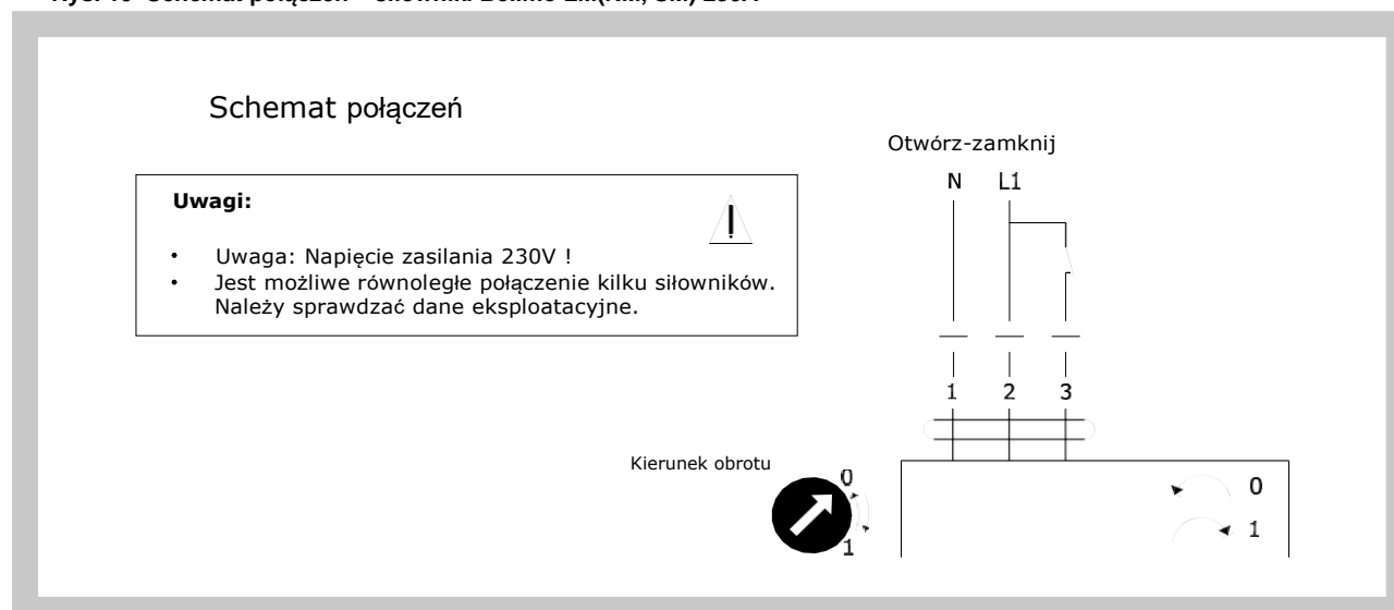
Rys. 10 Schemat połączeń – siłowniki Belimo LM(NM, SM) 230A
