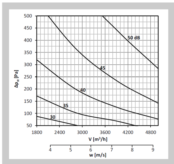
Diagram nr 67 Poziom mocy akustycznej LWA [dB(A)] na zewnątrz kanału 600x400, z izolacją
