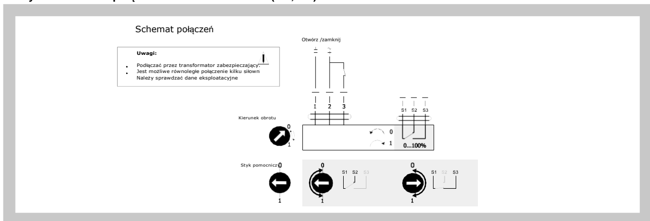
Rys. 14 Schemat połączeń – siłownik Belimo LM(NM, SM) 24A-S
