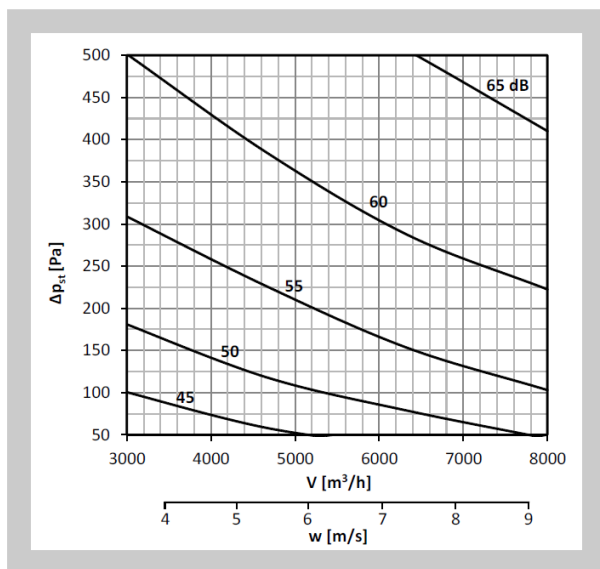
Diagram nr 46 Poziom mocy akustycznej LWA [dB(A)] na zewnątrz kanału 600x600, bez izolacji
