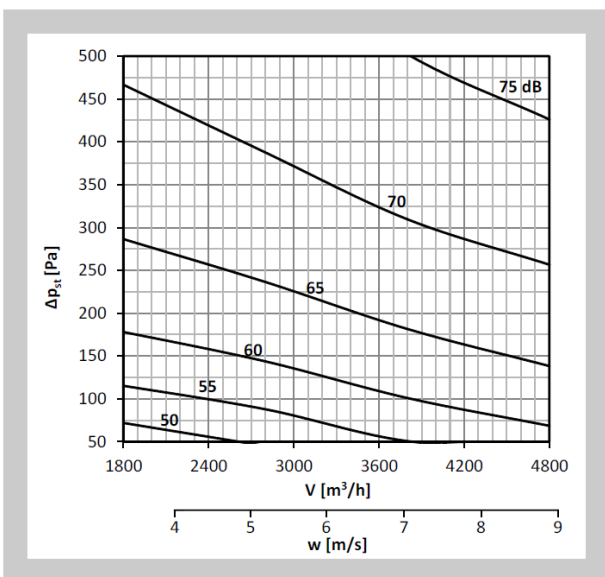
Diagram nr 17 Poziom mocy akustycznej L_{WA} [dB(A)] w kanale 500x500
