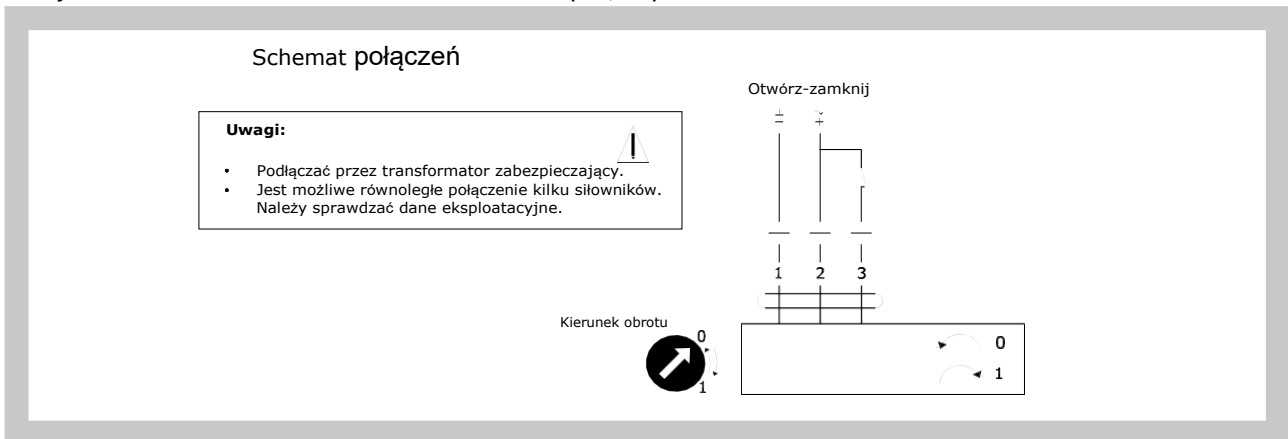
Rys. 12 Schemat połączeń - siłownik Belimo NM (SM) 24A-SR
