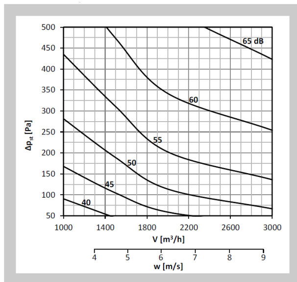
Diagram nr 33 Poziom mocy akustycznej LWA [dB(A)] na zewnątrz kanału 400x250, bez izolacji
