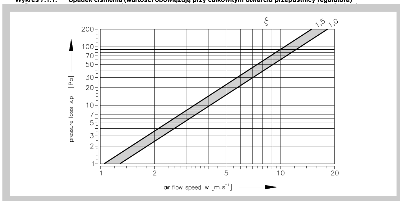
Wykres 7.1.1. Spadek ciśnienia (wartości obowiązują przy całkowitym otwarciu przepustnicy regulatora)
