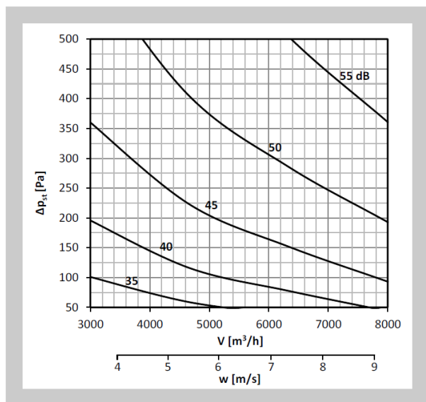
Diagram nr 69 Poziom mocy akustycznej LWA [dB(A)] na zewnątrz kanału 600x600, z izolacją
