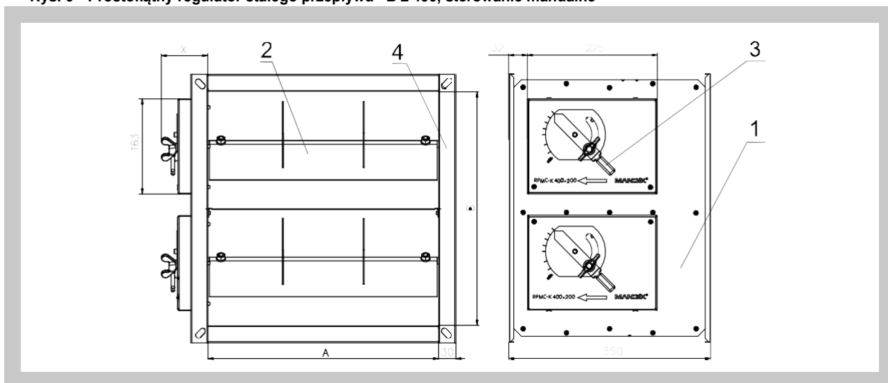
Rys. 6 Prostokątny regulator stałego przepływu - B ≥ 400, sterowanie manualne
