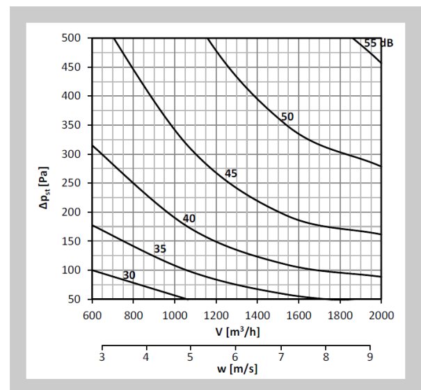
Diagram nr 52 Poziom mocy akustycznej LWA [dB(A)] na zewnątrz kanału 300x200, z izolacją
