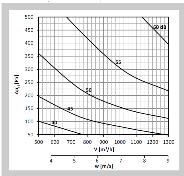
Diagram nr 28 Poziom mocy akustycznej LWA [dB(A)] na zewnątrz kanału 300x150, bez izolacji
