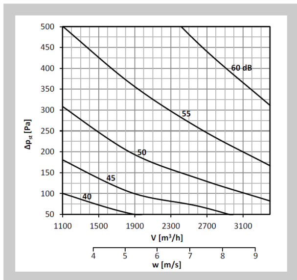
Diagram nr 38 Poziom mocy akustycznej LWA [dB(A)] na zewnątrz kanału 500x300, bez izolacji
