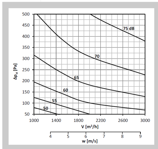
Diagram nr 10 Poziom mocy akustycznej L_{WA} [dB(A)] w kanale 400x250
