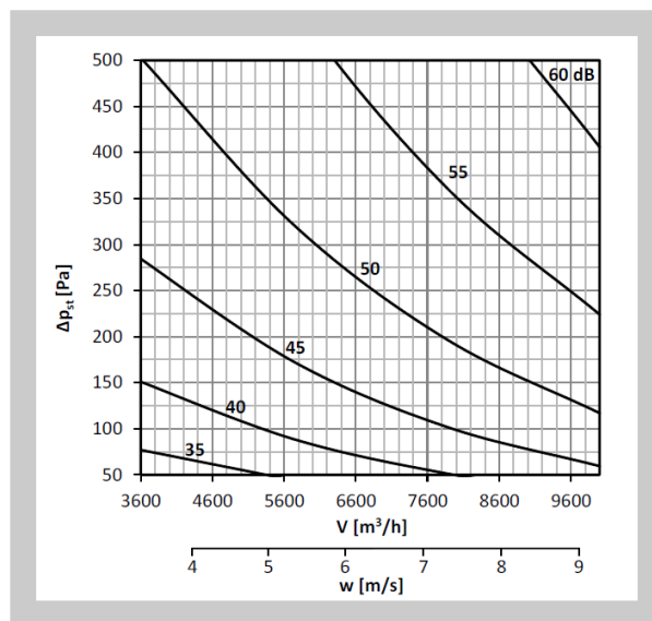
Diagram nr 68 Poziom mocy akustycznej LWA [dB(A)] na zewnątrz kanału 600x500, z izolacją
