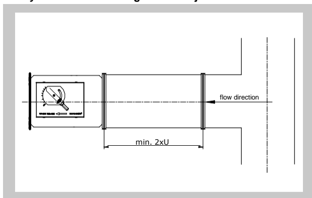
Rys. 7 Zalecana odległość od trójnika
