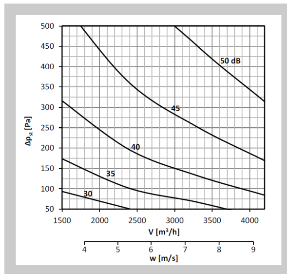
Diagram nr 62 Poziom mocy akustycznej LWA [dB(A)] na zewnątrz kanału 500x400, z izolacją
