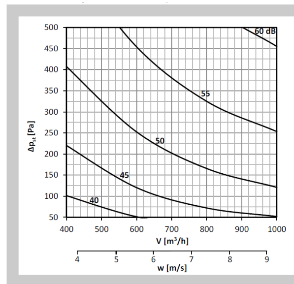
Diagram nr 29 Poziom mocy akustycznej LWA [dB(A)] na zewnątrz kanału 300x200, bez izolacji
