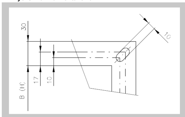
Rys. 9 Ramka montażowa
