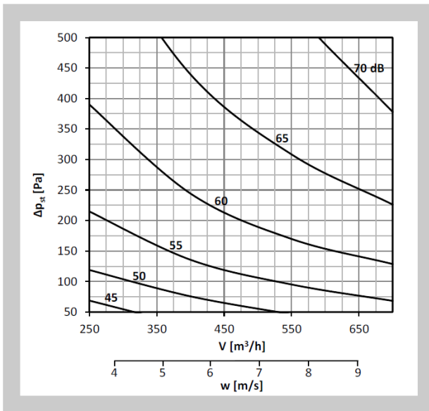
Diagram nr 3 Poziom mocy akustycznej L_{WA} [dB(A)] w kanale 200x200
