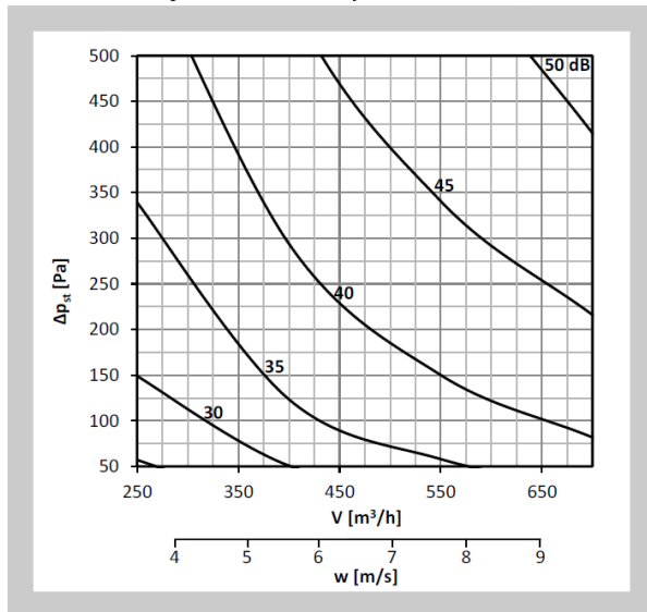
Diagram nr 49 Poziom mocy akustycznej LWA [dB(A)] na zewnątrz kanału 200x200, z izolacją
