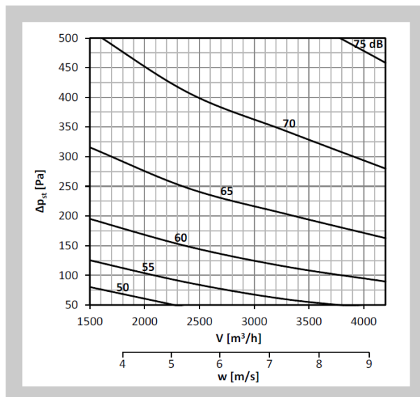
Diagram nr 16 Poziom mocy akustycznej L_{WA} [dB(A)] w kanale 500x400
