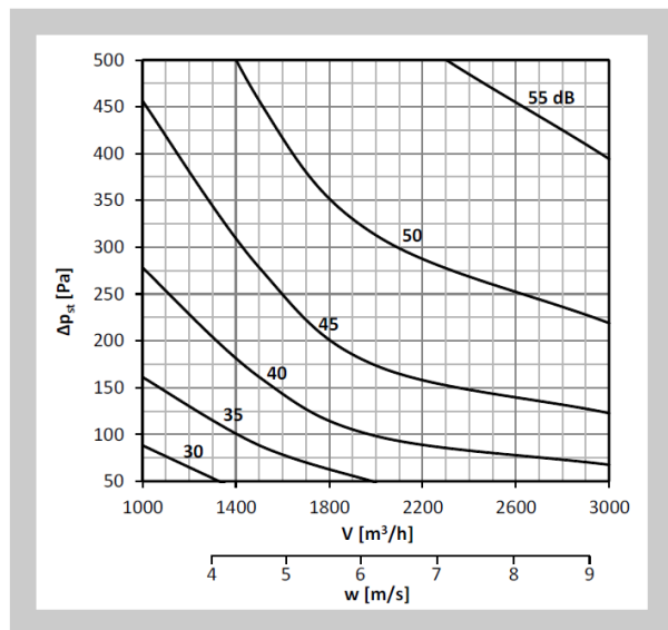
Diagram nr 56 Poziom mocy akustycznej LWA [dB(A)] na zewnątrz kanału 400x250, z izolacją
