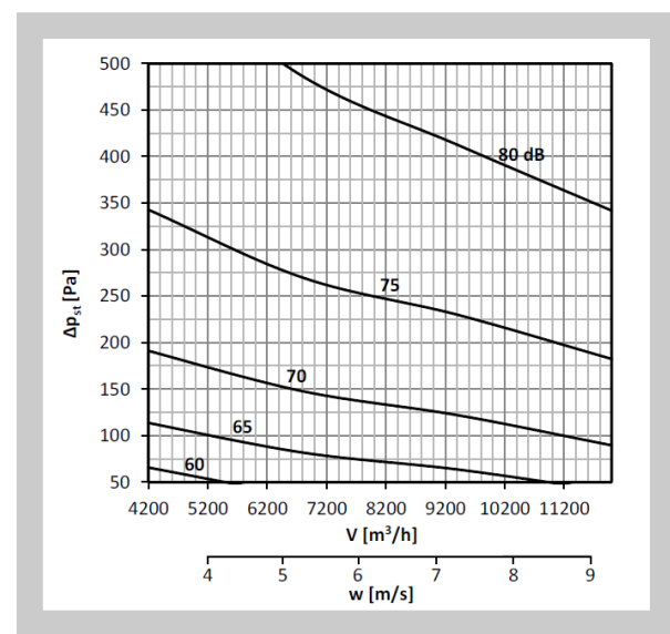
Diagram nr 23 Poziom mocy akustycznej L_{WA} [dB(A)] w kanale 600x600
