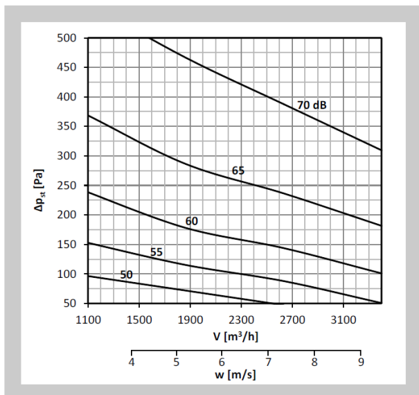
Diagram nr 15 Poziom mocy akustycznej L_{WA} [dB(A)] w kanale 500x300
