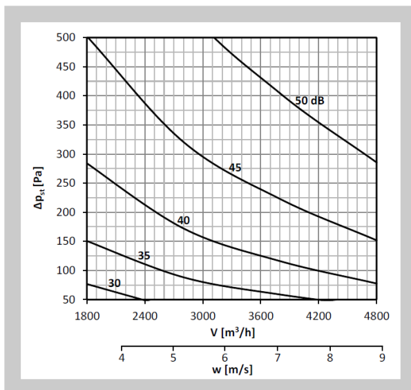
Diagram nr 63 Poziom mocy akustycznej LWA [dB(A)] na zewnątrz kanału 500x500, z izolacją
