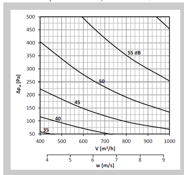
Diagram nr 27 Poziom mocy akustycznej LWA [dB(A)] na zewnątrz kanału 300x100, bez izolacji
