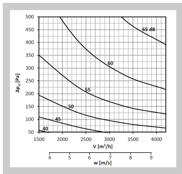
Diagram nr 34 Poziom mocy akustycznej LWA [dB(A)] na zewnątrz kanału 400x300, bez izolacji
