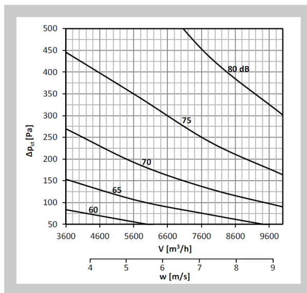
Diagram nr 22 Poziom mocy akustycznej L_{WA} [dB(A)] w kanale 600x500
