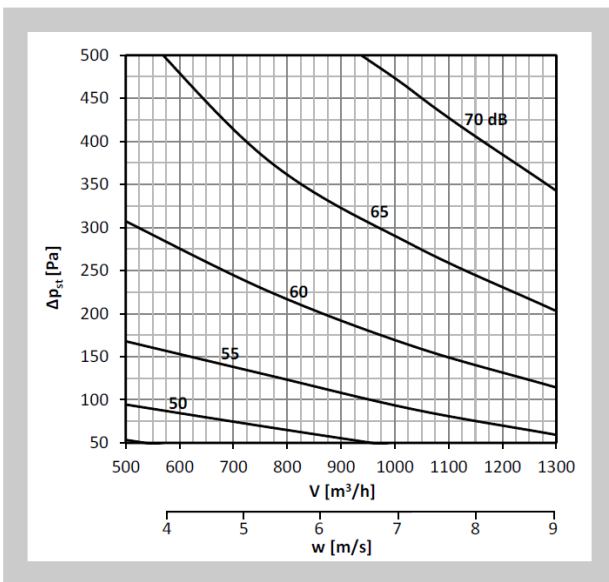
Diagram nr 5 Poziom mocy akustycznej L_{WA} [dB(A)] w kanale 300x150
