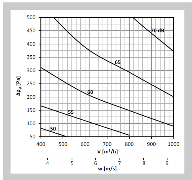
Diagram nr 6 Poziom mocy akustycznej L_{WA} [dB(A)] w kanale 300x200
