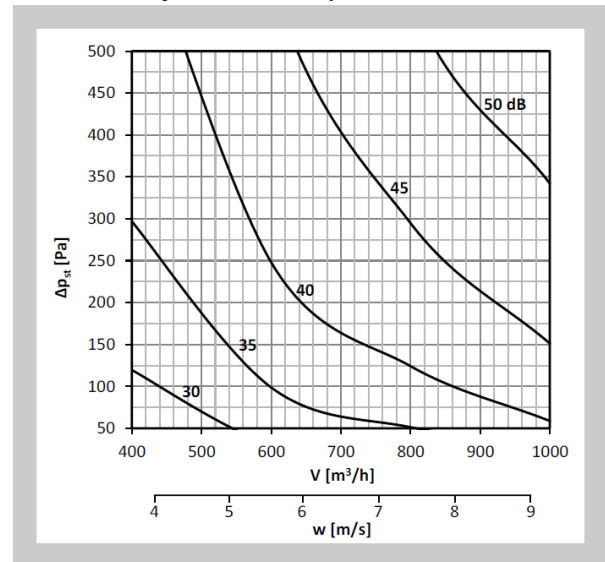
Diagram nr 50 Poziom mocy akustycznej LWA [dB(A)] na zewnątrz kanału 300x100, z izolacją
