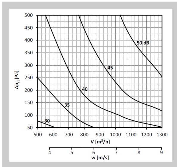
Diagram nr 51 Poziom mocy akustycznej LWA [dB(A)] na zewnątrz kanału 300x150, z izolacją
