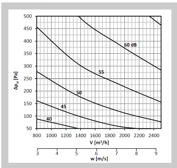
Diagram nr 32 Poziom mocy akustycznej LWA [dB(A)] na zewnątrz kanału 400x200, bez izolacji
