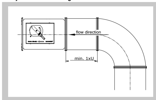
Rys. 8 Zalecana odległość od kolana
