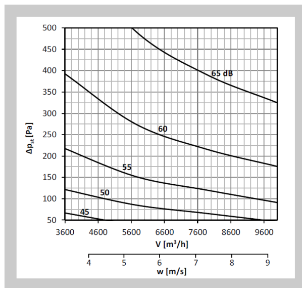
Diagram nr 45 Poziom mocy akustycznej LWA [dB(A)] na zewnątrz kanału 600x500, bez izolacji
