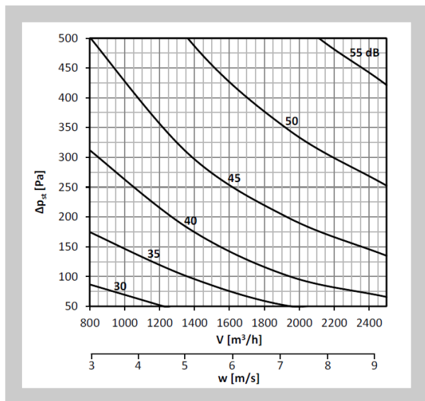
Diagram nr 55 Poziom mocy akustycznej LWA [dB(A)] na zewnątrz kanału 400x200, z izolacją
