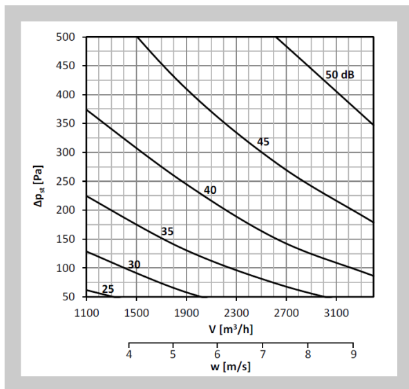
Diagram nr 61 Poziom mocy akustycznej LWA [dB(A)] na zewnątrz kanału 500x300, z izolacją
