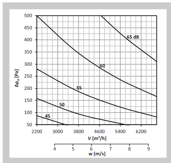
Diagram nr 41 Poziom mocy akustycznej LWA [dB(A)] na zewnątrz kanału 600x200, bez izolacji
