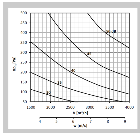
Diagram nr 64 Poziom mocy akustycznej LWA [dB(A)] na zewnątrz kanału 600x200, z izolacją
