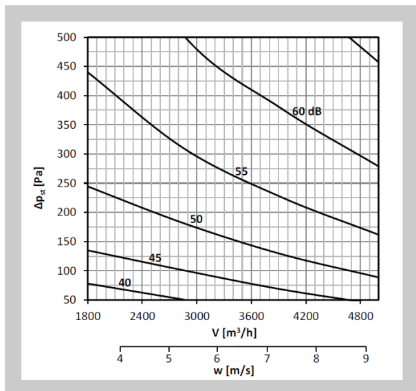
Diagram nr 44 Poziom mocy akustycznej LWA [dB(A)] na zewnątrz kanału 600x400, bez izolacji
