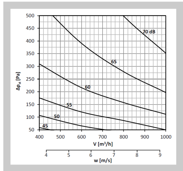
Diagram nr 4 Poziom mocy akustycznej L_{WA} [dB(A)] w kanale 300x100
