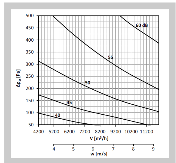
Diagram nr 69 Poziom mocy akustycznej LWA [dB(A)] na zewnątrz kanału 600x600, z izolacją
