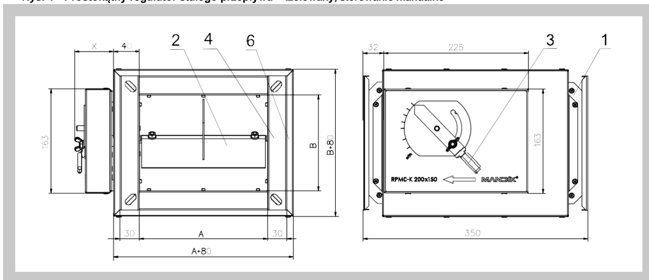
Rys. 5 Prostokątny regulator stałego przepływu - sterowanie siłownikiem
