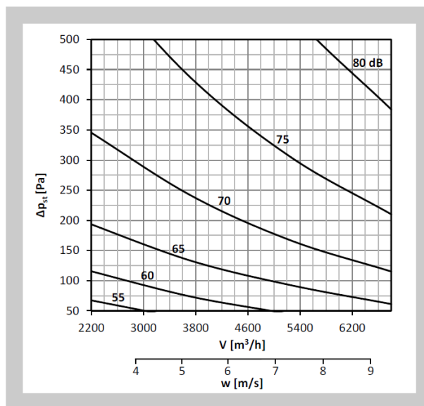
Diagram nr 18 Poziom mocy akustycznej L_{WA} [dB(A)] w kanale 600x200
