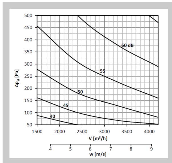
Diagram nr 39 Poziom mocy akustycznej LWA [dB(A)] na zewnątrz kanału 500x400, bez izolacji
