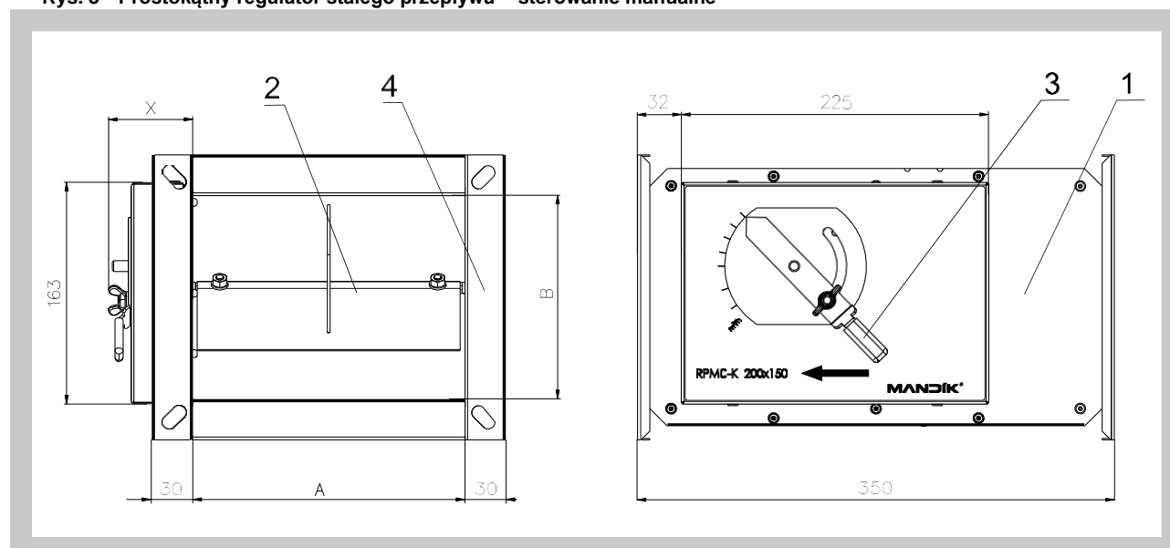
Rys. 3 Prostokątny regulator stałego przepływu - sterowanie manualne
