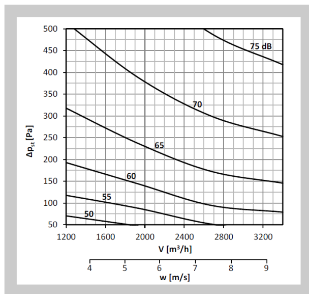
Diagram nr 12 Poziom mocy akustycznej L_{WA} [dB(A)] w kanale 400x400
