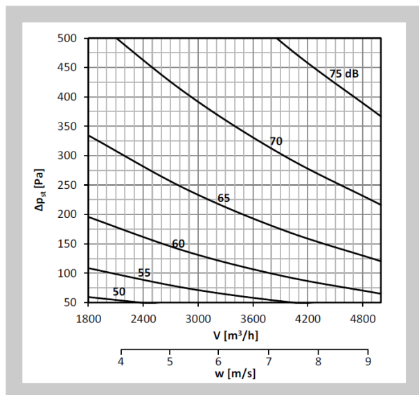
Diagram nr 21 Poziom mocy akustycznej L_{WA} [dB(A)] w kanale 600x400
