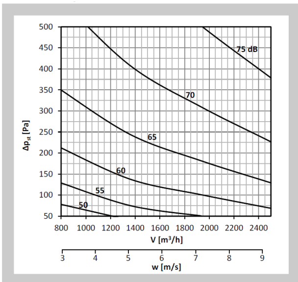
Diagram nr 9 Poziom mocy akustycznej L_{WA} [dB(A)] w kanale 400x200
