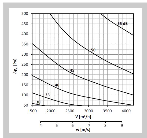
Diagram nr 57 Poziom mocy akustycznej LWA [dB(A)] na zewnątrz kanału 400x300, z izolacją
