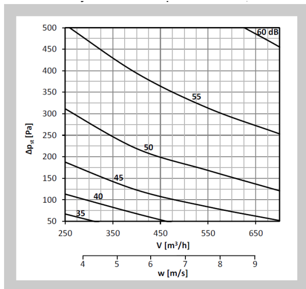
Diagram nr 26 Poziom mocy akustycznej LWA [dB(A)] na zewnątrz kanału 200x200, bez izolacji
