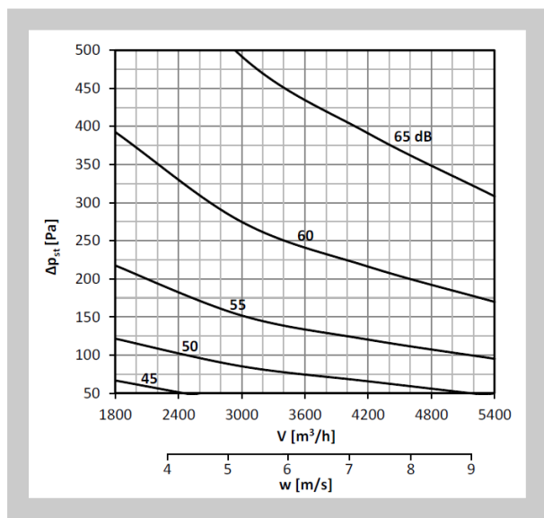
Diagram nr 35 Poziom mocy akustycznej LWA [dB(A)] na zewnątrz kanału 400x400, bez izolacji
