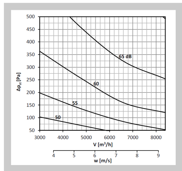
Diagram nr 40 Poziom mocy akustycznej LWA [dB(A)] na zewnątrz kanału 500x500, bez izolacji
