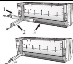
Łączenie rurki przyłączeniowej
